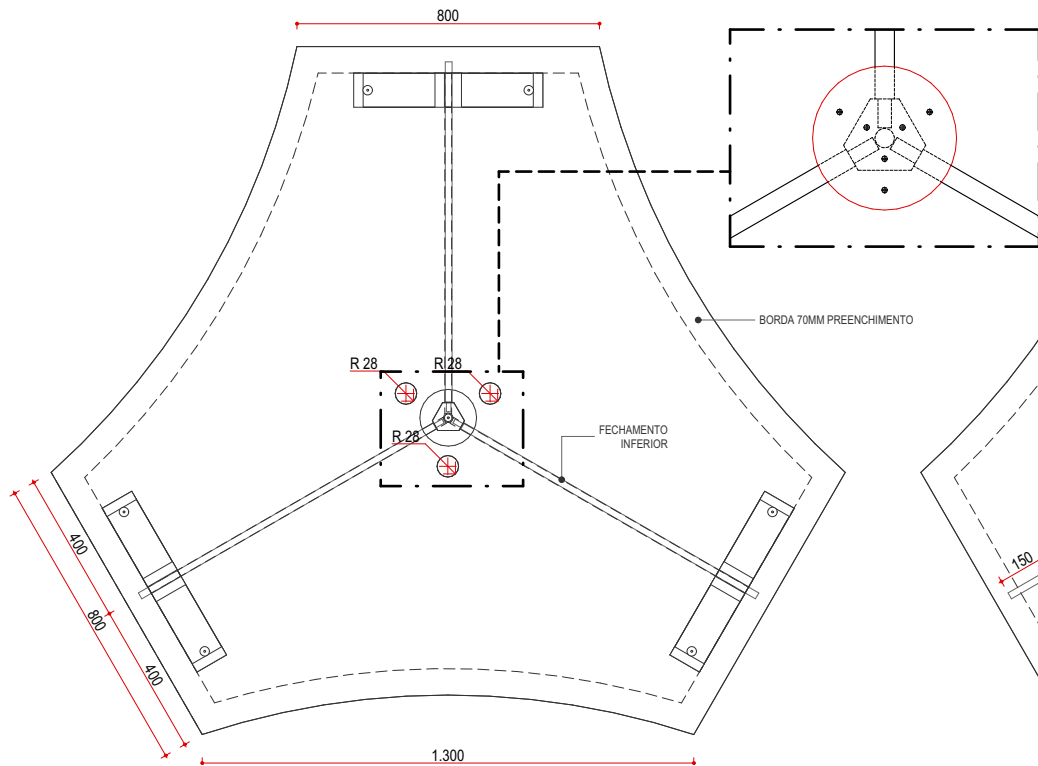
VISTA SUPERIOR
