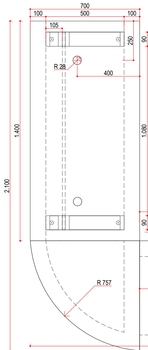
VISTA SUPERIOR
