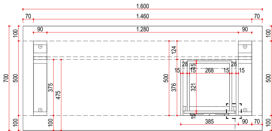
DETALHE
