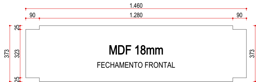
DETALHE
