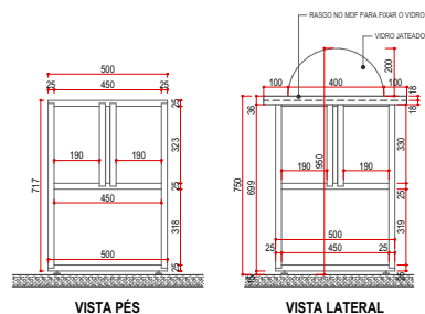
VISTA PÉS
